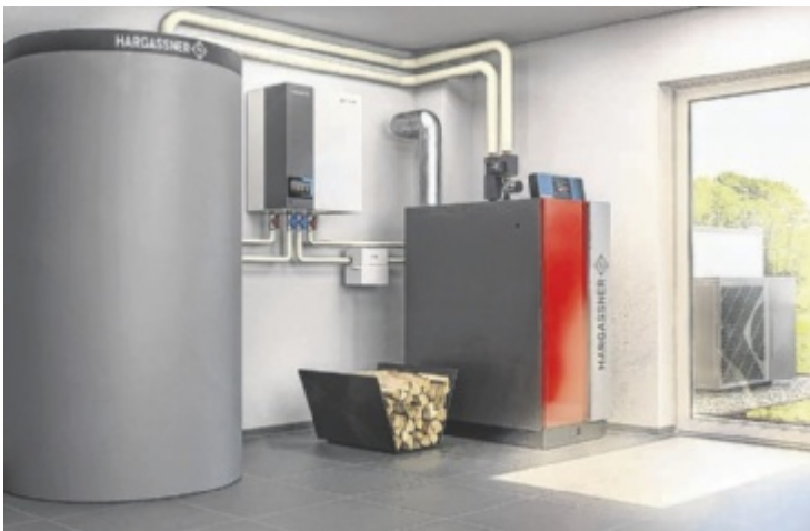
Eine Wärmepumpe lässt sich zum Beispiel mit einem Biomassekessel kombinieren, der nur bei höherem Bedarf eingesetzt wird.
