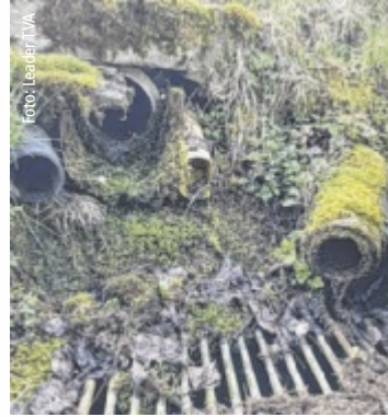
Ein einfaches Drainagesystem schützt Hänge vor Abschwemmung.
