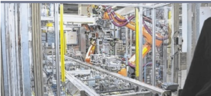
Zweite Linie Seit August läuft im BMW Werk Steyr die Serienproduktion der E-Motoren für den neuen, vollelektrischen BMW iX3. Jetzt startet man mit einer zweiten E-Linie in die Vorserie. Details: www.tips.at/n/703972 Foto: BMW Group
