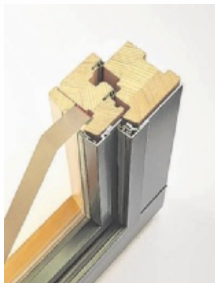
Fensterprofil aus Aluminium
